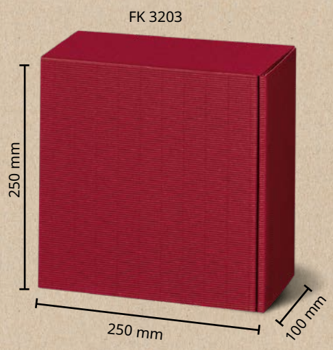
VARIO BOX NR. 3 OFFENE WELLE 250 x 250 x 100 mm, VE = 25 St. FK 3203 - Bordeaux, innen bordeaux FK 3204 - Anthrazit, innen anthrazit
