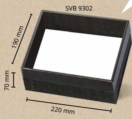
VARIO BODEN OFFENE WELLE MINI UND TRANSPARENTER DECKEL Bodenteil ohne Einlage, innen weiss 220 x 190 x 70 mm, VE = 25 St. SVB 9302 - Bodenteil, schwarz SVB 9300 - Bodenteil, natur Deckel: SVD 9200 - Deckel, transparent BODENTEIL UND DECKEL MÜSSEN SEPARAT BESTELLT WERDEN
