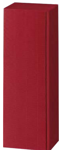
CHAMPAGNER OFFENE WELLE BORDEAUX für extra breite Flaschen bis max. Ø 100 mm, Innenseite + Einlage bordeaux, Einlage offene Welle, nicht DHL-zertifiziert, VE = 50 St. WK 31301 - 1 x 0,75 l, 317 x 100 x 100 mm
